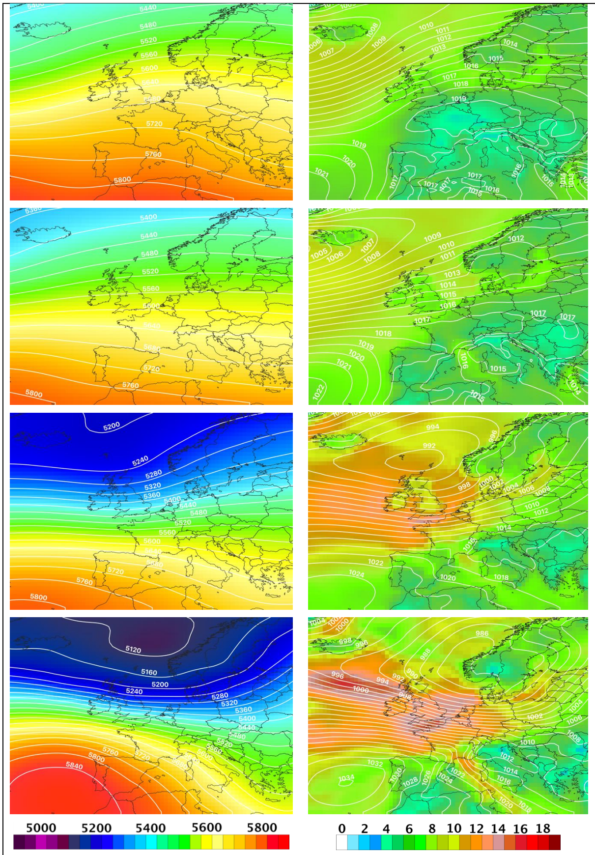
Figure 1. Configurations moyennes du géopotiel 500hPa en mètres à gauche, et de la pression atmosphérique en hPa et de la vitesse du vent en surface en m/s à droite pour les classes 0-10%, 20-30%, 60-70% et 80-90% de facteur de charge de l'éolien en France de 2012 à 2018.
