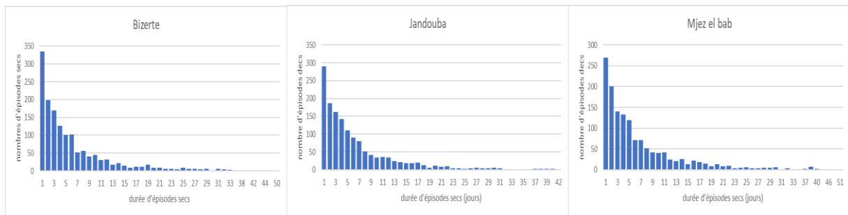
Figure 2. Durée des épisodes secs dans le grenier de la Tunisie (plaine de Bizerte ; moyenne vallée de Mejerda(Jandouba et Mjez el bab) de 1970-71 à 2014-15.
